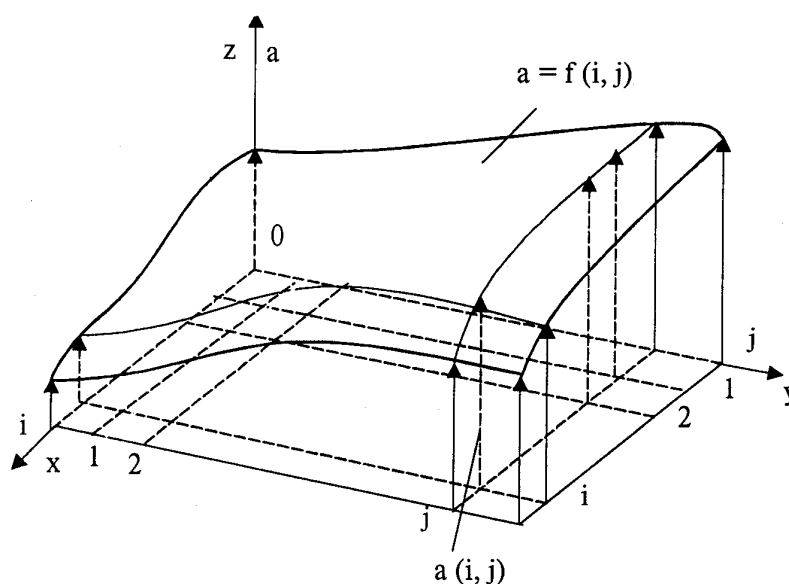
Геометрическое представление матрицы поверхностью в трехмерном пространстве
