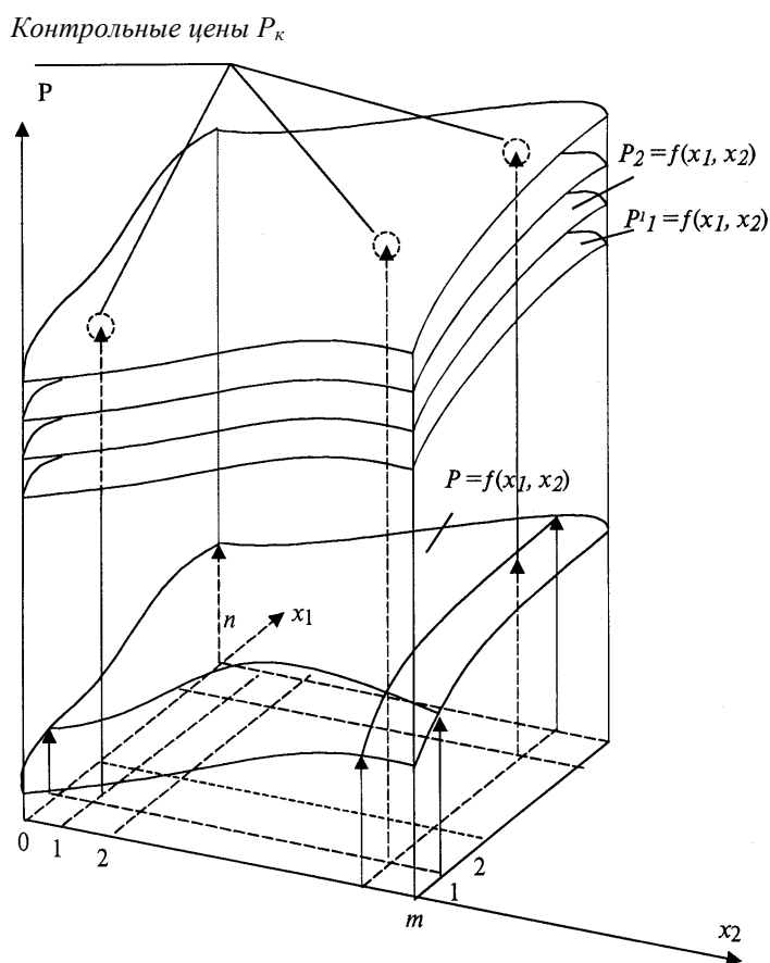
Геометрическая объемная интерпретация прейскуранта цен поверхностью P = f(x_1, x_2) в трехмерном пространстве (параметрическая модель рынка товаров группового ассортимента – «этажерка» цен)
